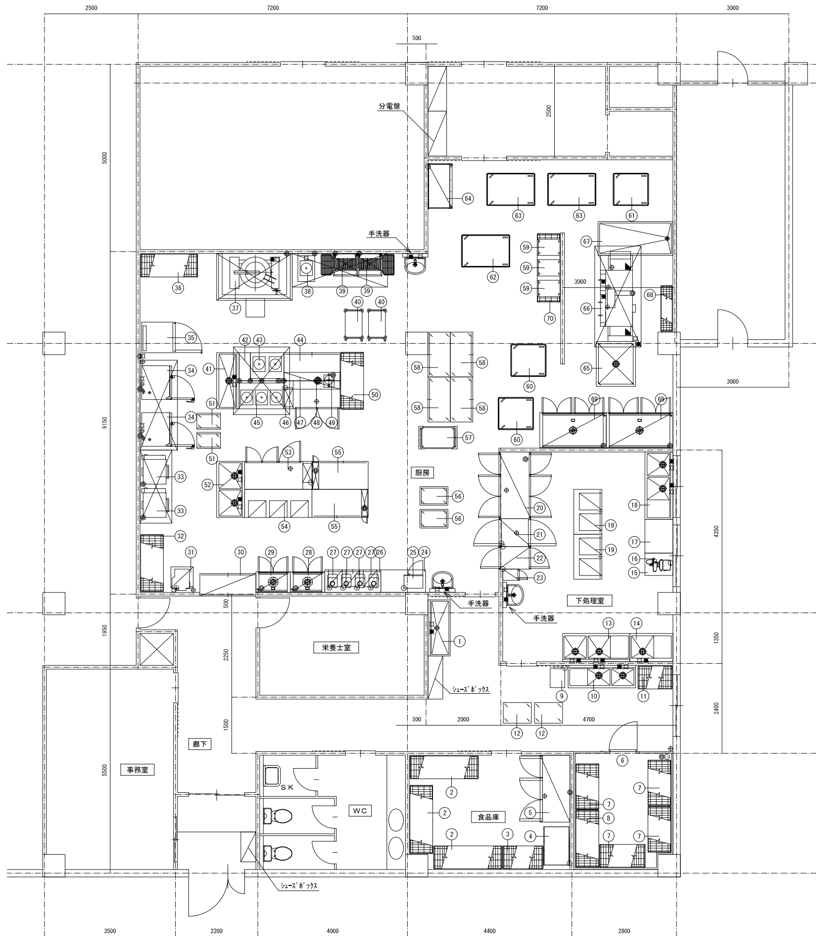
厨房レイアウト参考図 S=1:50 A3縮小版はS=1:100
