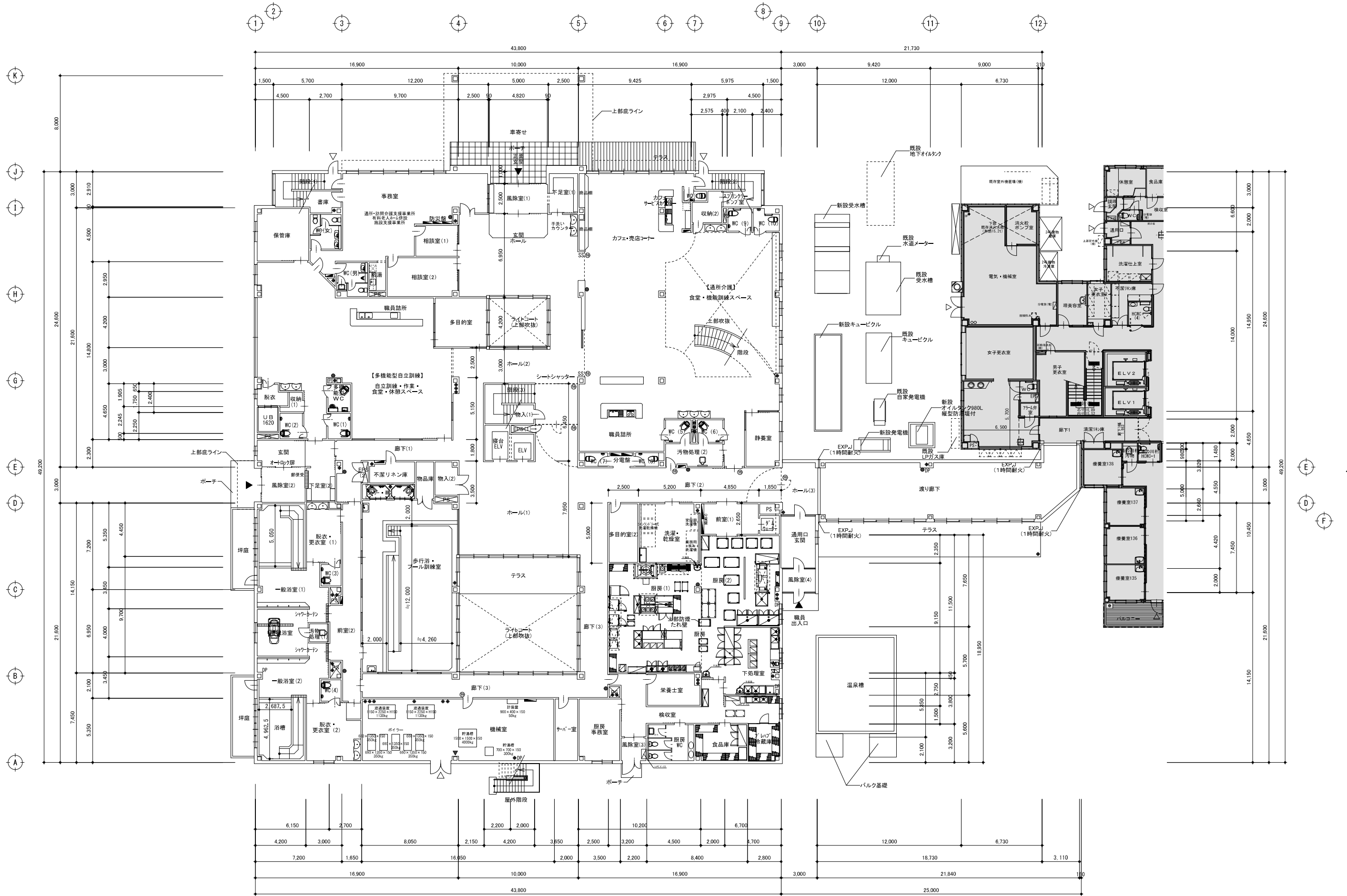
1階平面図 S=1:300
